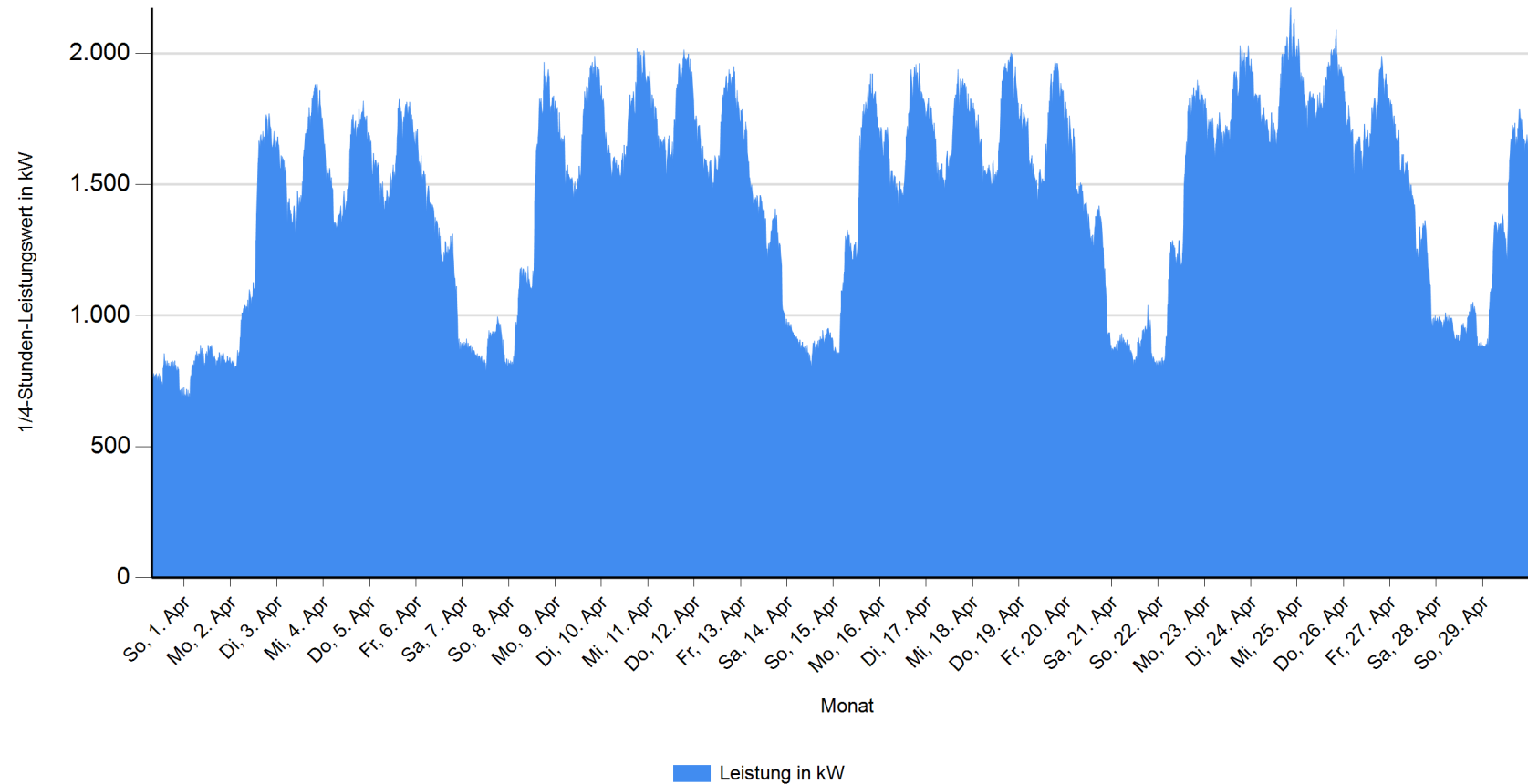
Grafische Darstellung eines Monatslastganges
