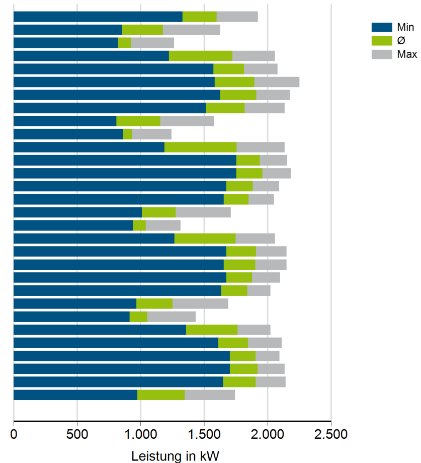
Verteilung der Leistungswerte im Monat
